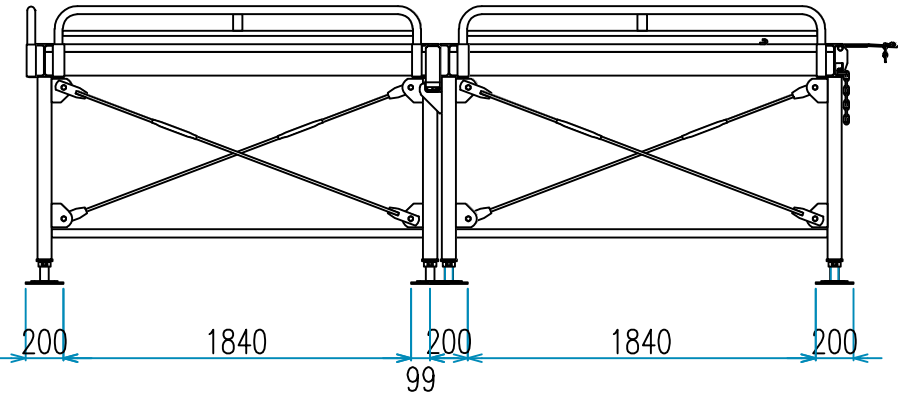
架台1-2
